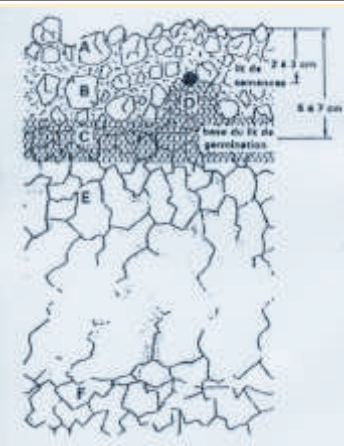
Figure 1: Schéma du lit de semence recherché pour la culture de la betterave monogermine (ITB, 1992)
